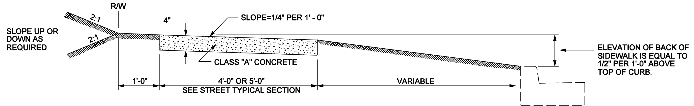
SECTION A-A
