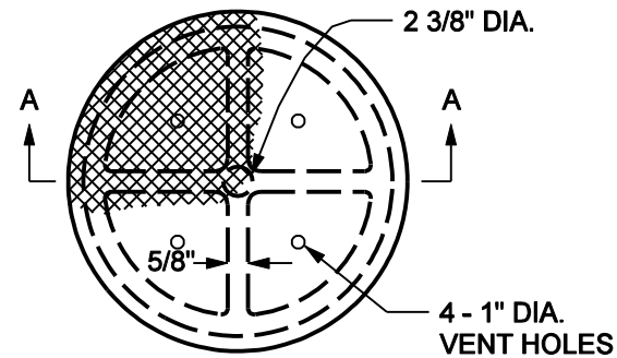
PLAN MANHOLE LID
