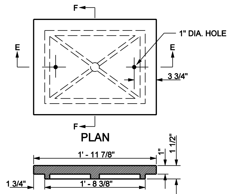
SECTION E - E LID
