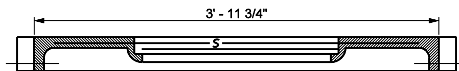
SECTION C - C FRAME MIN. WT. - 215 LBS.
