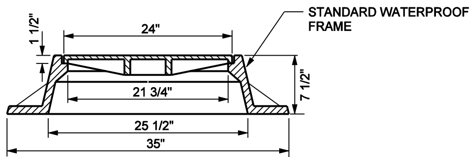
SECTION - FRAME & LID
